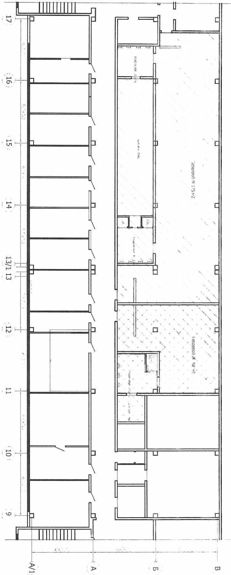
План на отг. +3,600 2 ЭТАЖ
